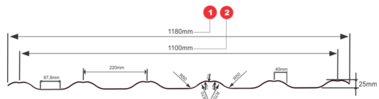
1 - Обща ширина 2 - Ефективна ширина
